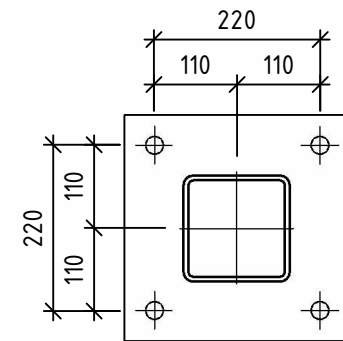
FÖRSTÖRING 1 : 10 GRUNDBULTAR
